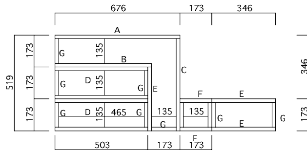
正面図
