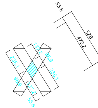
足・・・合いカギ部分寸法
